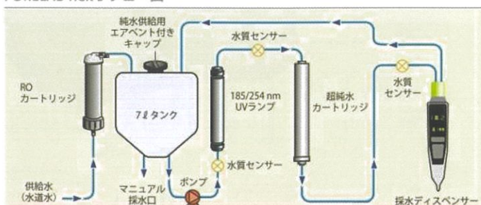
PURELAB flex3 フロー図
