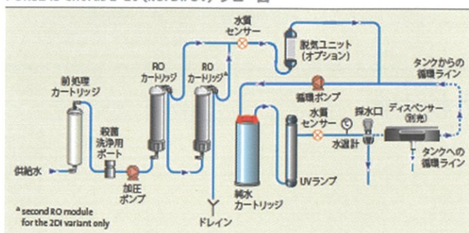
PURELAB Chorus 2+ 20 (RO/DI/UV) フロー図
